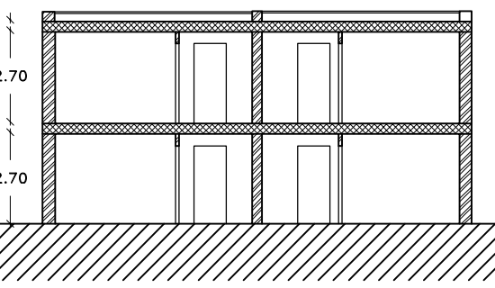
SEZIONE X-Y
