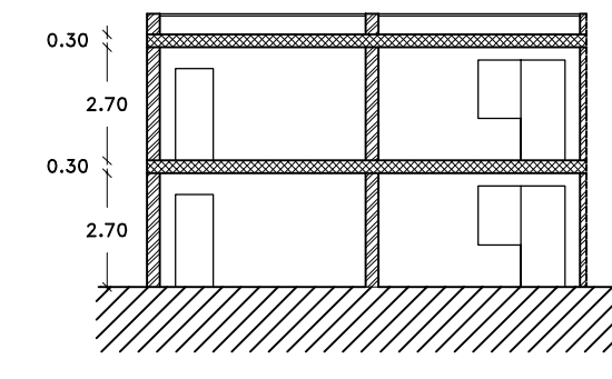
SEZIONE X-Y
