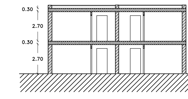
SEZIONE X-Y
